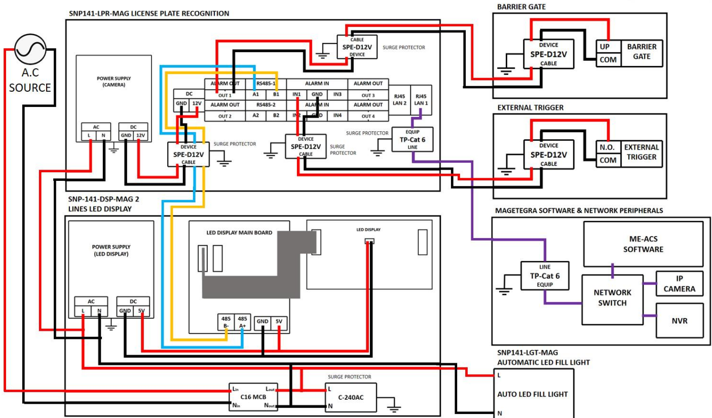
Fig. 21: Wiring Diagram
